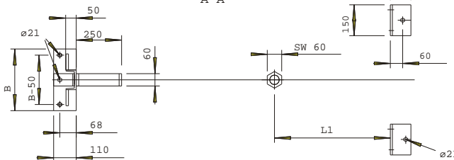
Anschlussvarianten DIN 2501
