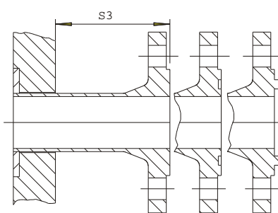
Connections DIN 2501
