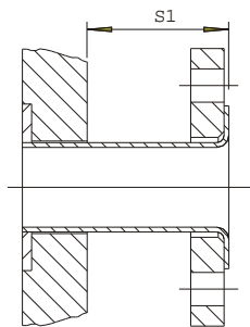
Anschlussvarianten DIN 2501
