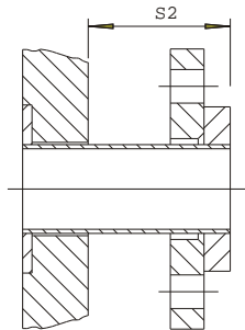
Anschlussvarianten DIN 2501
